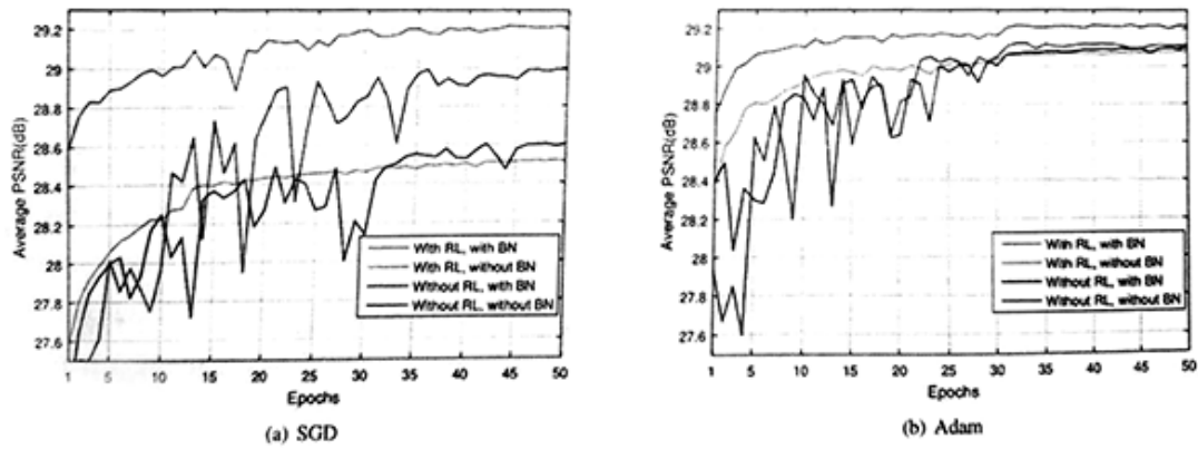
Рис. 2 – Использование алгоритмов оптимизации
