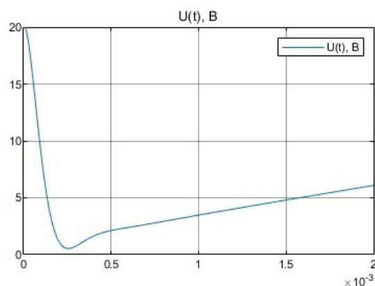
Рис. 1 – Переходный процесс на выходе РТ без компенсации ЭДС вращения ЭД
