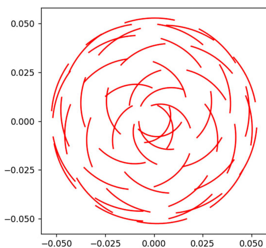
Рис. 4 – Визуализация движения лазера по гипотрохоидной траектории скорости движения луча 5 мм/с.
