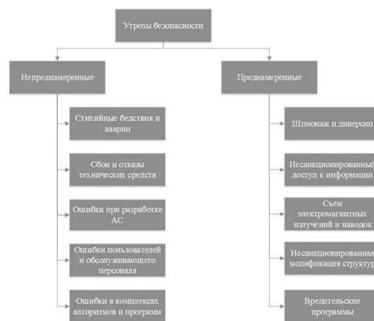
Рис. 1 – Угрозы кибербезопасности
